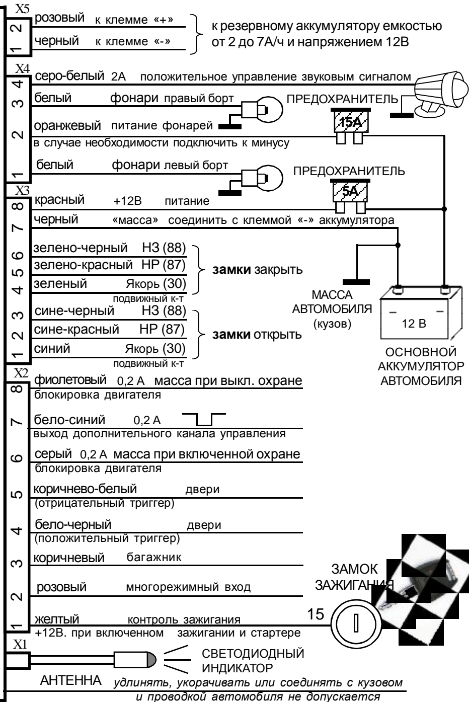
Рис. Схема основных подключений.
