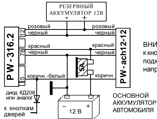
Рис.3. Подключение резервного аккумулятора и контроллера заряда PW-ach12-12.
